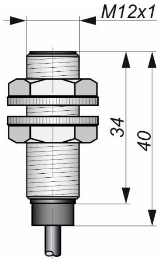
Габаритный чертеж
